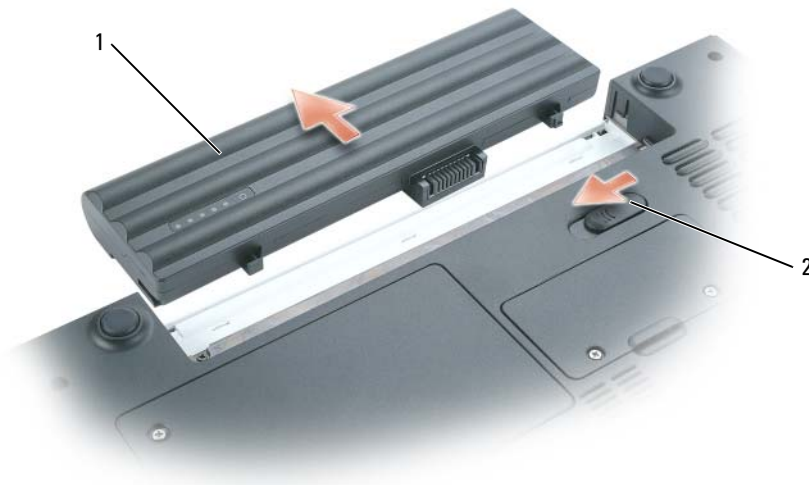
1 電池
