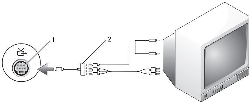
1 S-video 電視輸出連接器 2 元件影像配接器
