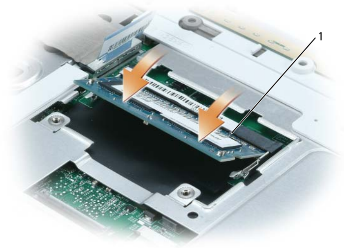
1 連接器插槽中的彈片
