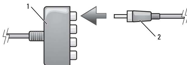
1 元件影像配接器 2 S/PDIF 數位音效纜線
