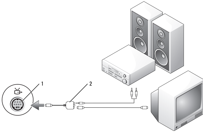
1 S-video 電視輸出連接器 2 合成式影像配接器
