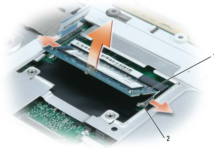
1 記憶體模組
