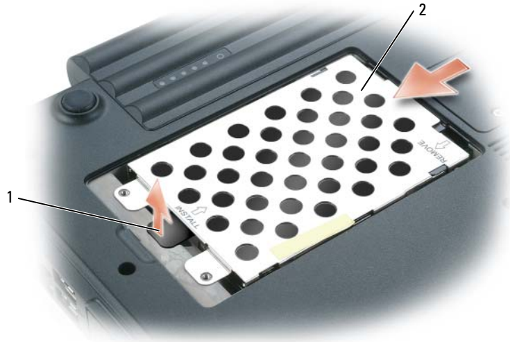
1 拉式彈片
