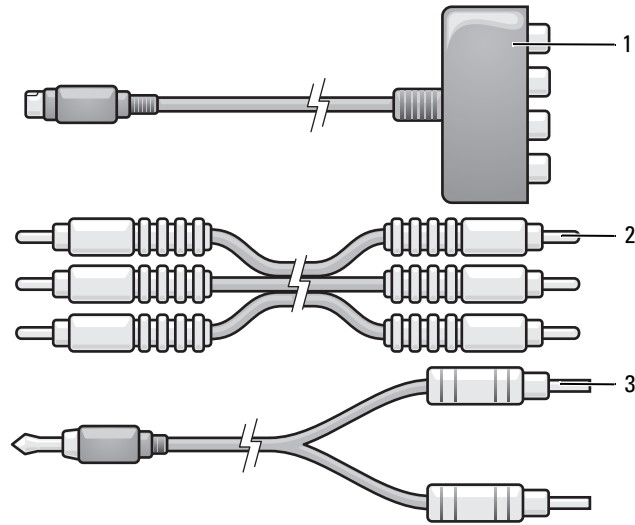
1 元件影像配接器 2 元件影像纜線 3 標準音效纜線
